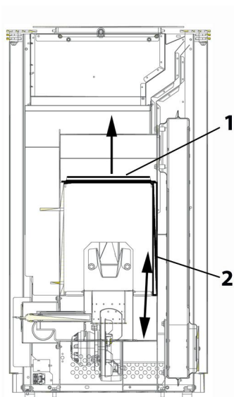
Obr. 8a: Demontáž deflektoru (clony)
