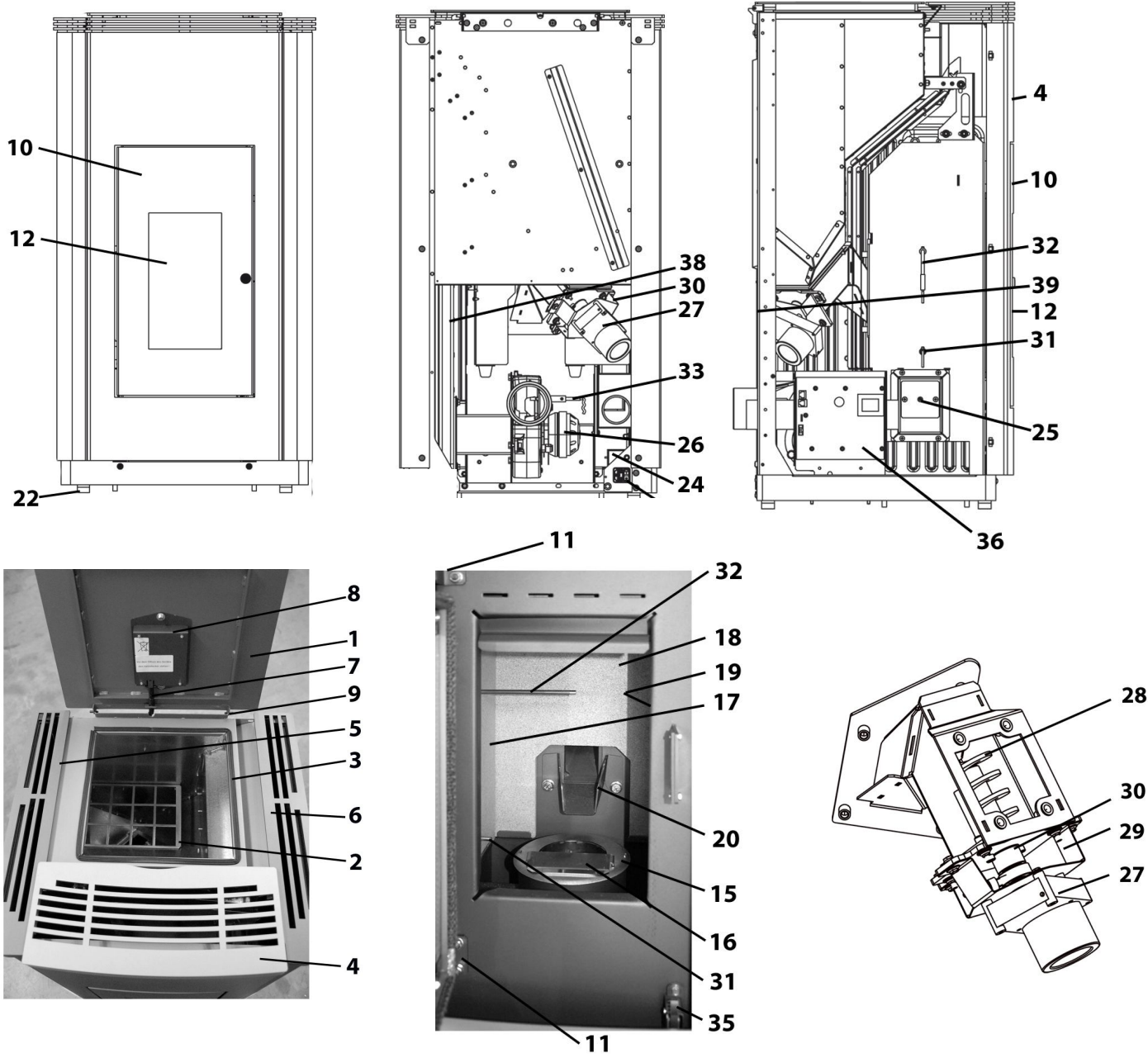
Obrázky 23: Náhradní díly 417.08
