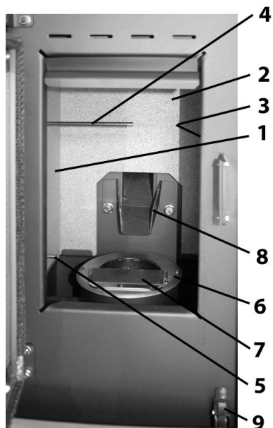
Obrázek 17: Prostor topeniště
