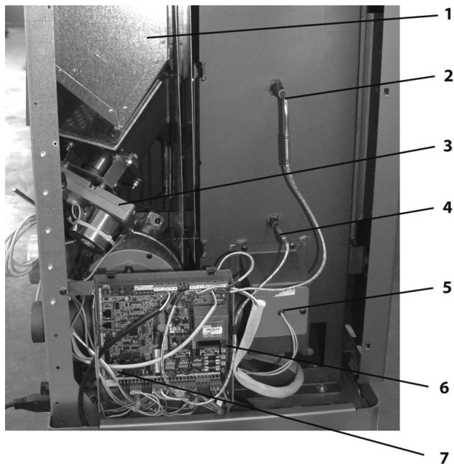
Obrázek 12: Elektrické součásti
